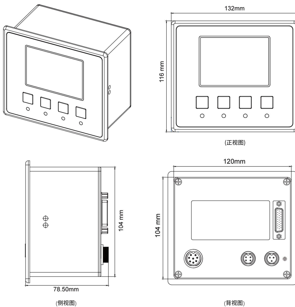
图 1-1: 主机尺寸图
