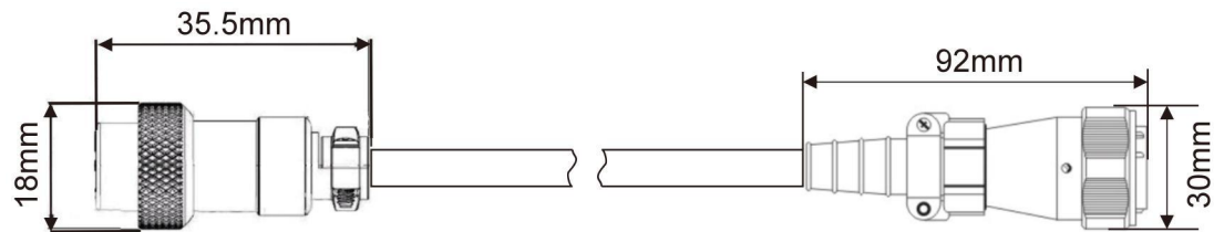
图 1-5：传感器电缆尺寸图
