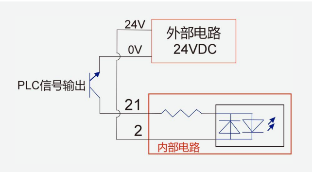
图 2-9：测量输入 IO 与 PLC 接线图
