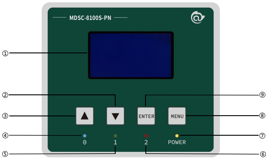
图 2-1：主机面板示意图
