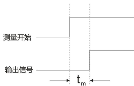
图 2-11：测量时间说明
