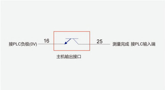
图 2-10：测量完成输出 IO 与 PLC 接线图
