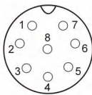
图 2-5：传感器脚位示意图
