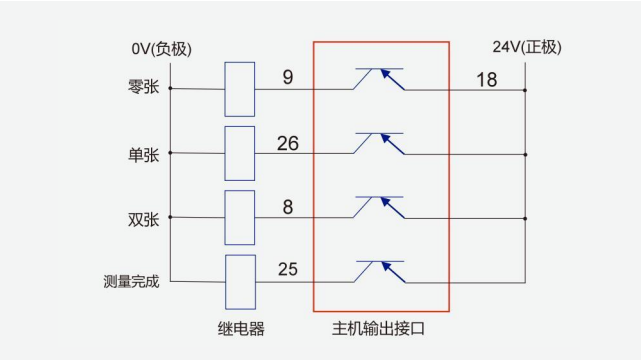
图 2-7：主机输出接口与继电器接线图
