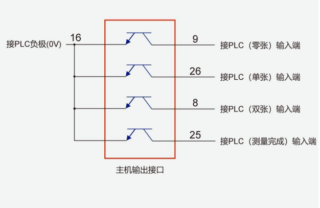
图 2-8：主机输出接口与 PLC 接线图
