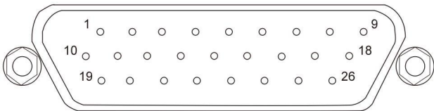
图 2-6：输入输出接口示意图
