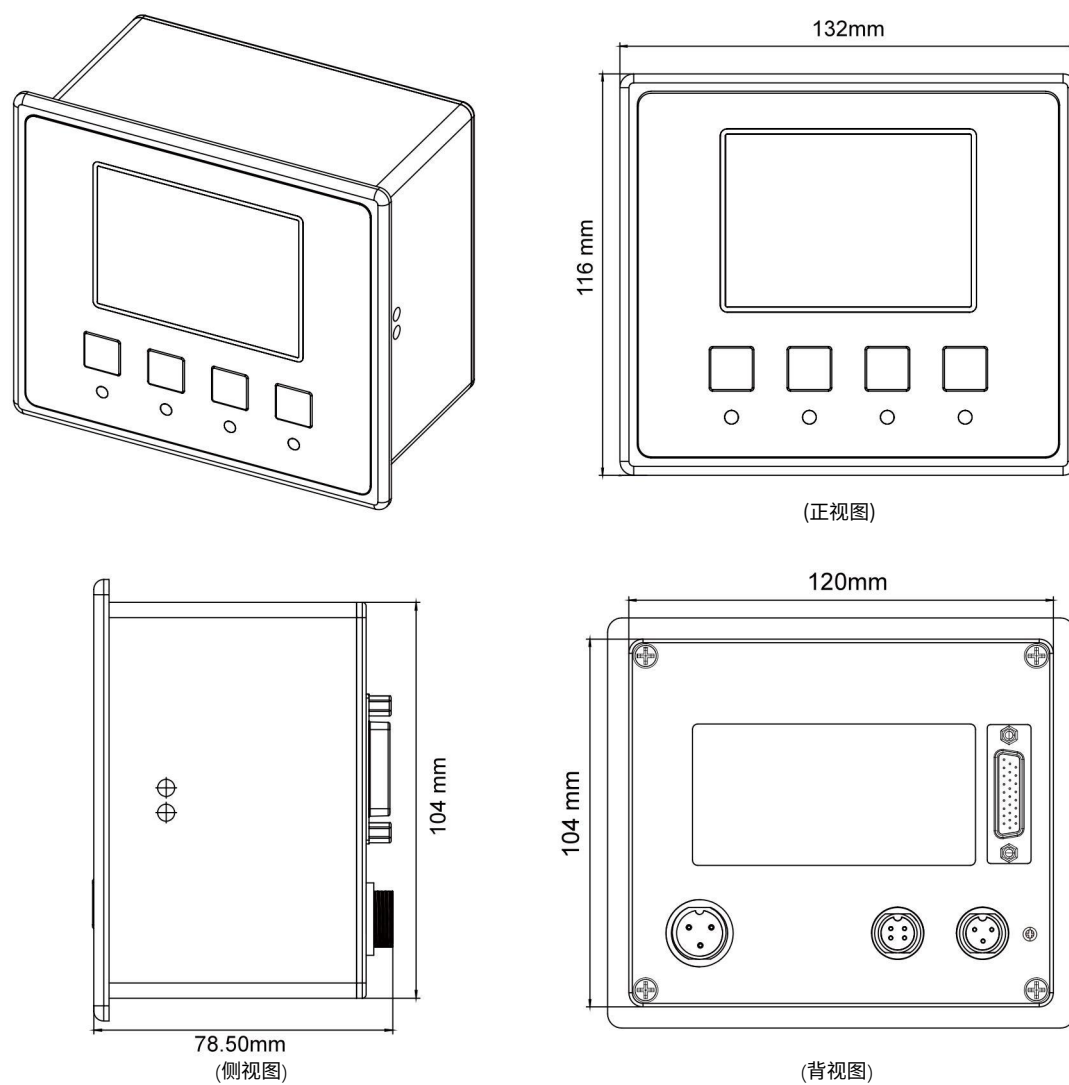
图 1-1: 主机尺寸图
