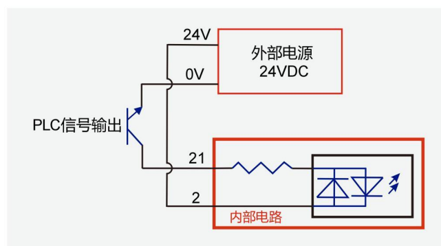
NPN
