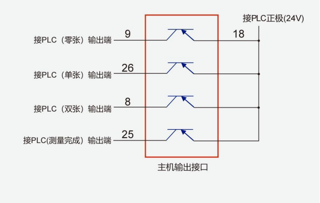
图 2-8：主机输出接口与 PLC 接线图
