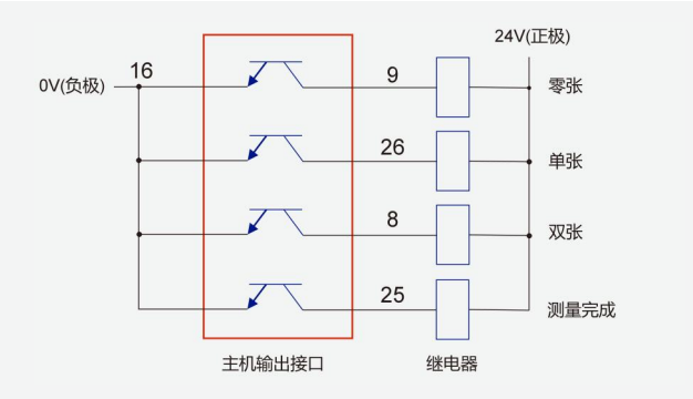
图 2-7：主机输出接口与继电器接线图
