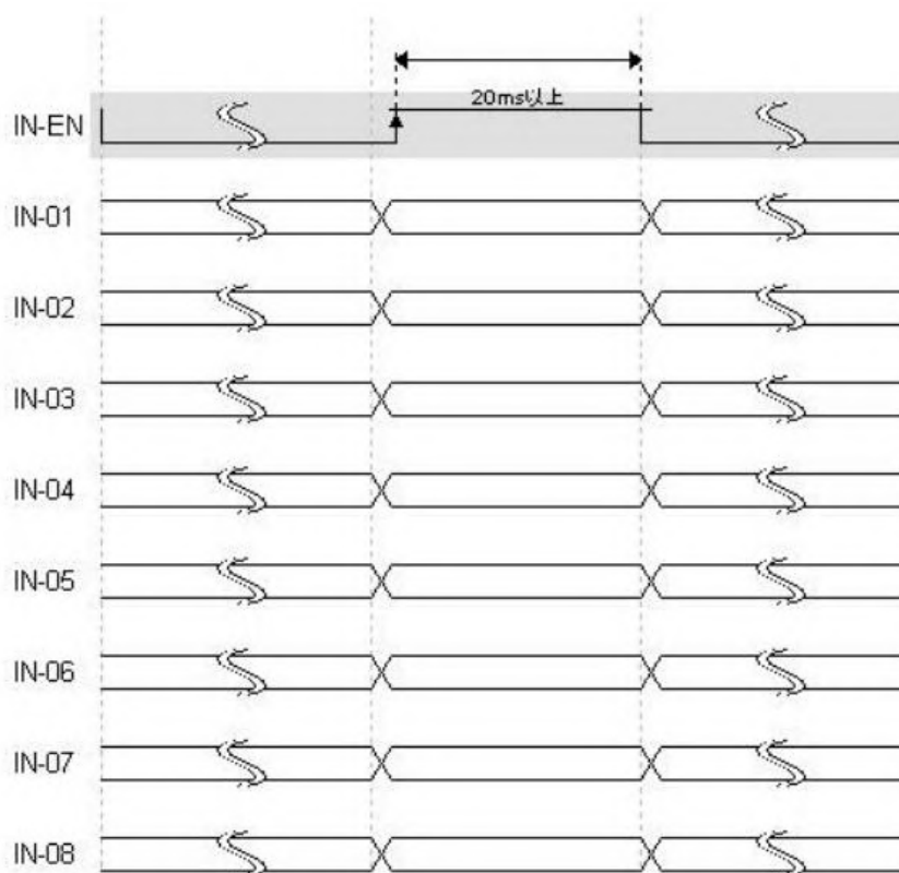
图 4-1：外部 IO 切换控制时序图
