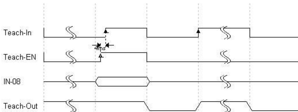
图 4-2：外部示教时序图
