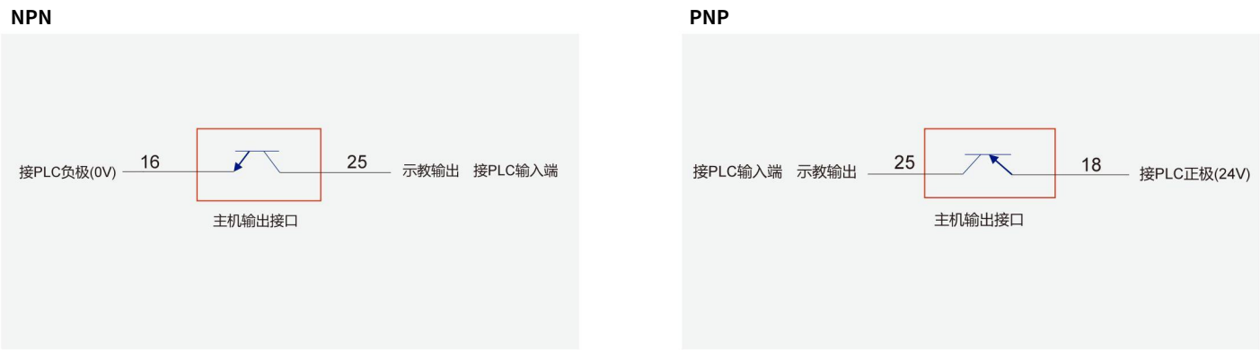
图 2-10：示教输出 IO 与 PLC 接线图
