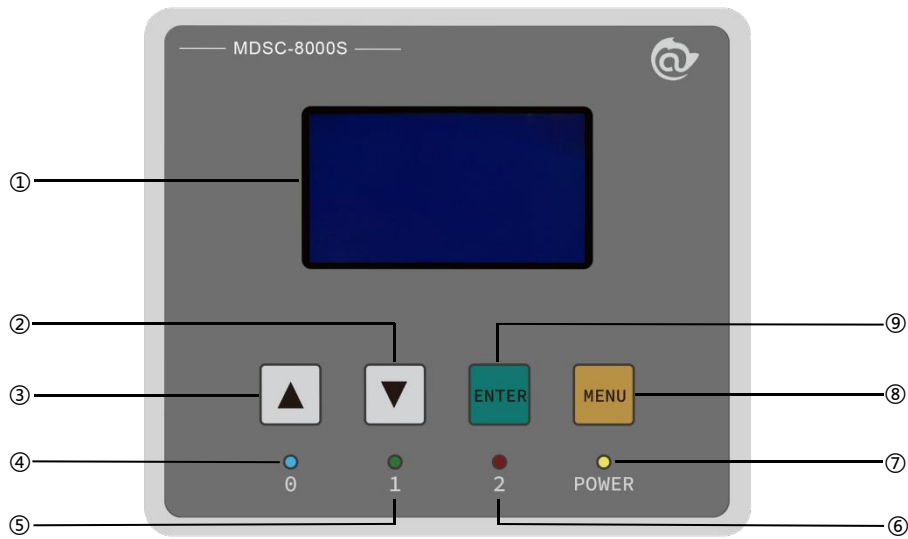
2-1：主机面板示意图
