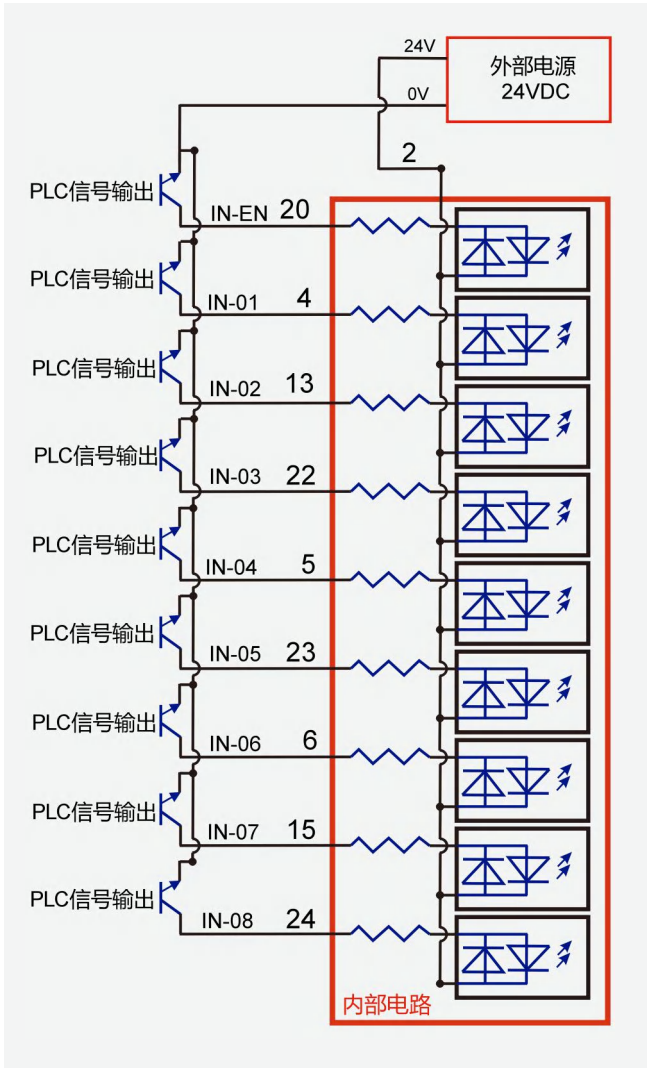
NPN
