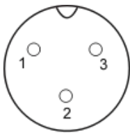
图 2-5：传感器脚位示意图
