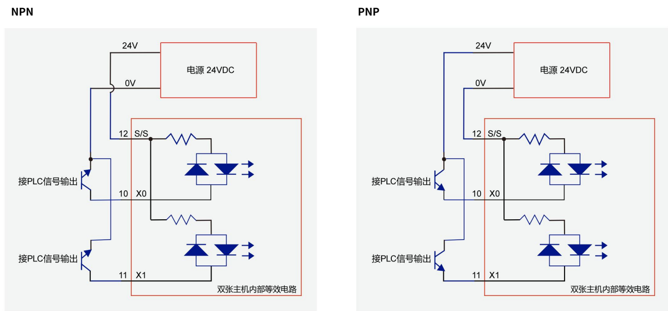
图 3-6：记忆组切换 IO 输入接线图
