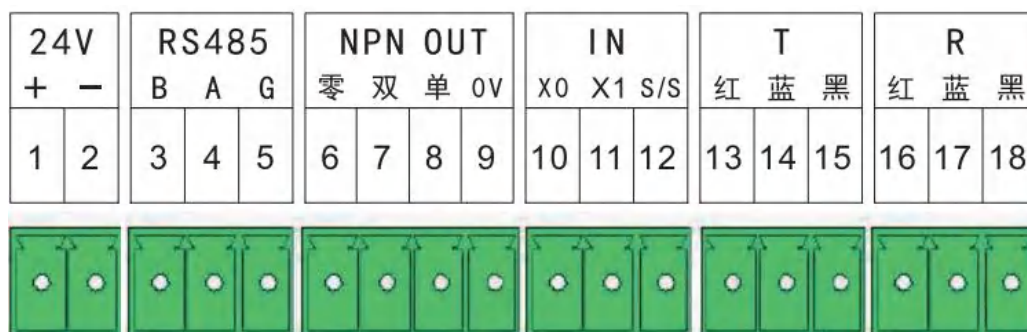
图 3-2：NPN 接线说明
