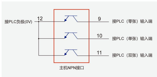
图 3-5：主机输出接口与 PLC 接线图
