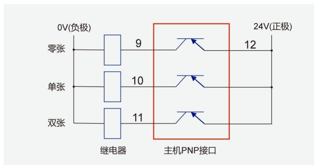
图 3-4：主机输出接口与继电器接线图
