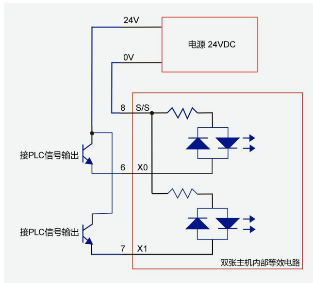
图 3-6：记忆组切换 IO 输入接线图
