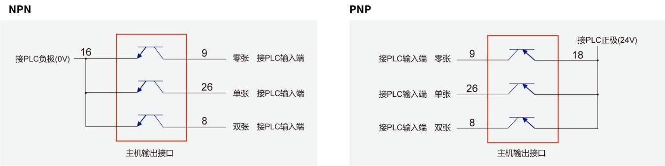
图 2-7：主机输出接口与 PLC 接线图
