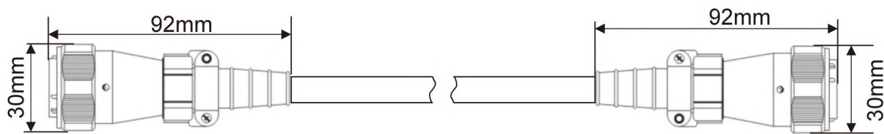
图 1-5：传感器电缆尺寸图
