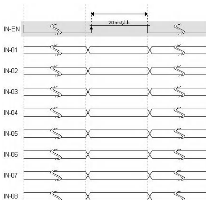
图 4-1: 外部 IO 切换控制时序图
