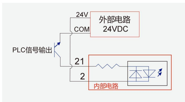
图 2-11：测量使能信号与 PLC 接线图
