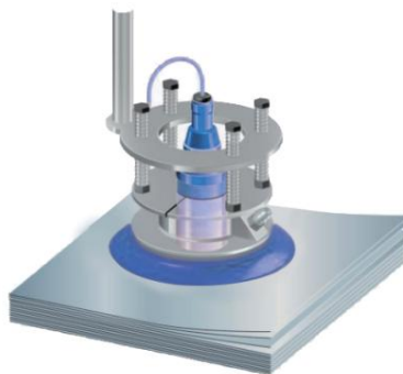
图 3-1：传感器安装示意图
