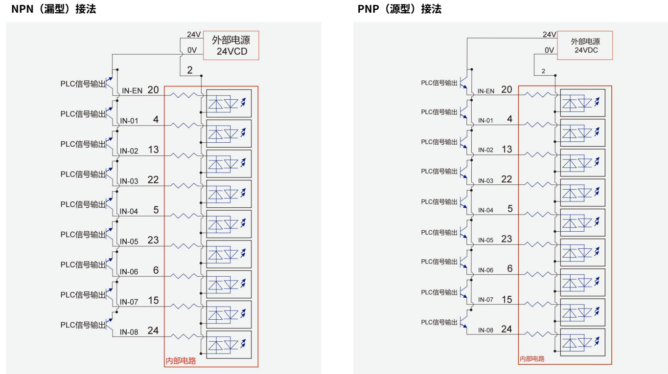
图 2-8：外部 IO 选择片料接口与 PLC 接线图
