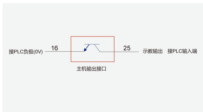
图 2-10：示教输出 IO 与 PLC 接线图
