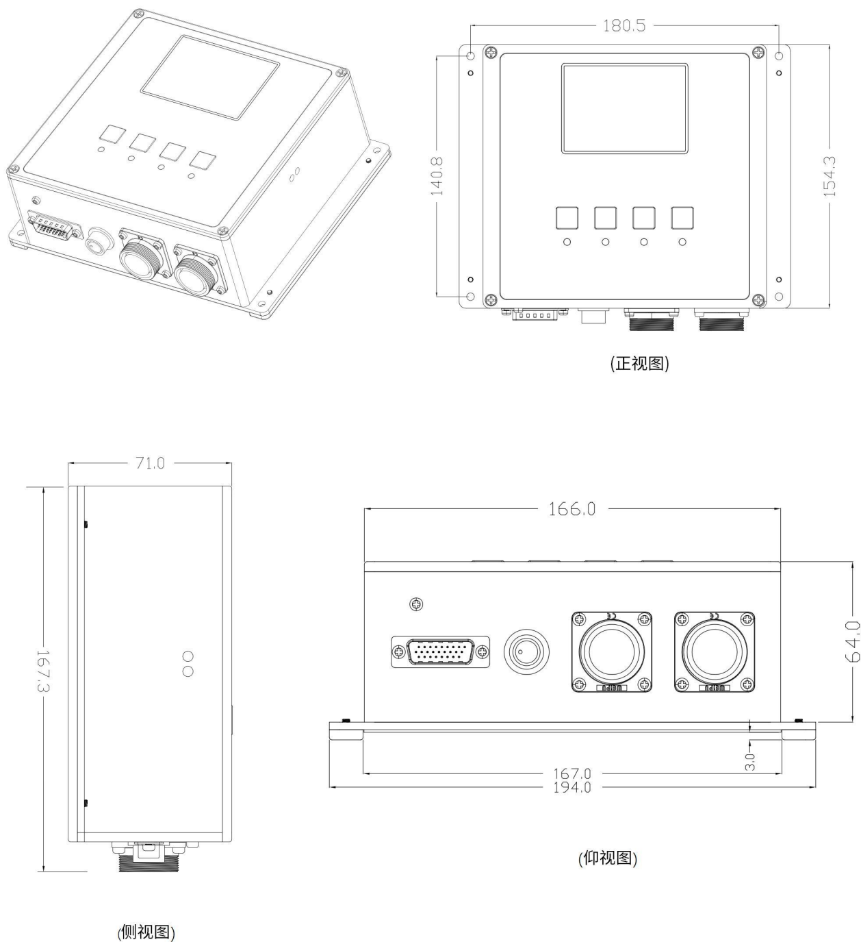
图 1-2: 主机尺寸图 (底座安装式)
