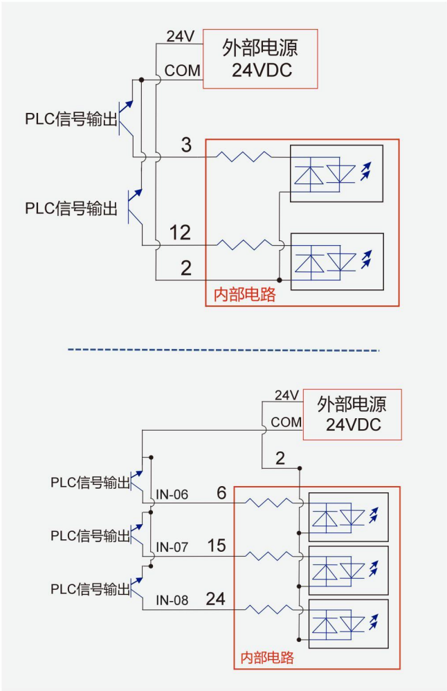
图 2-9：示教输入 IO 与 PLC 接线图
