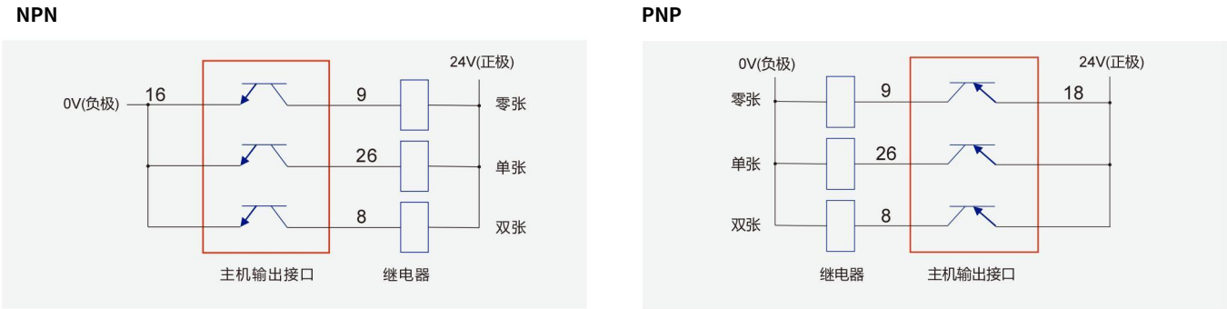
图 2-6：主机输出接口与继电器接线图
