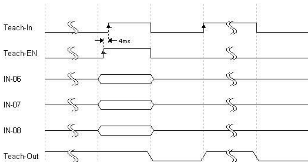
图 4-2：外部示教时序图
