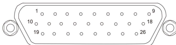
图 2-3: 输入输出接口示意图
