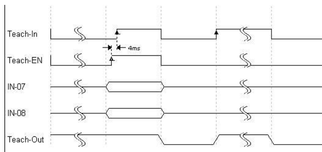
图 4-2：外部示教时序图
