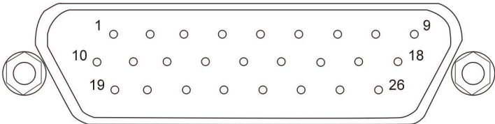
图 2-6: 输入输出接口示意图
