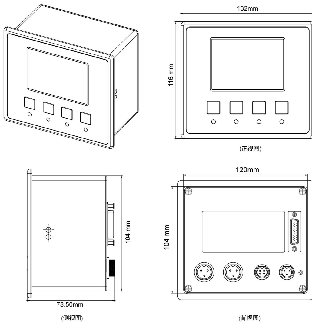
图 1-1: 主机尺寸图
