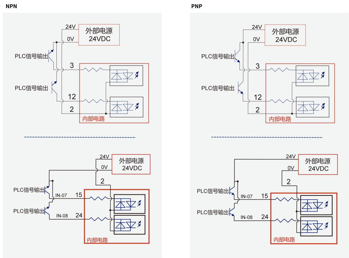
图 2-9：示教输入 IO 与 PLC 接线图
