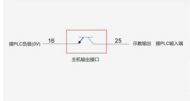
图 2-11：示教输出 IO 与 PLC 接线图
