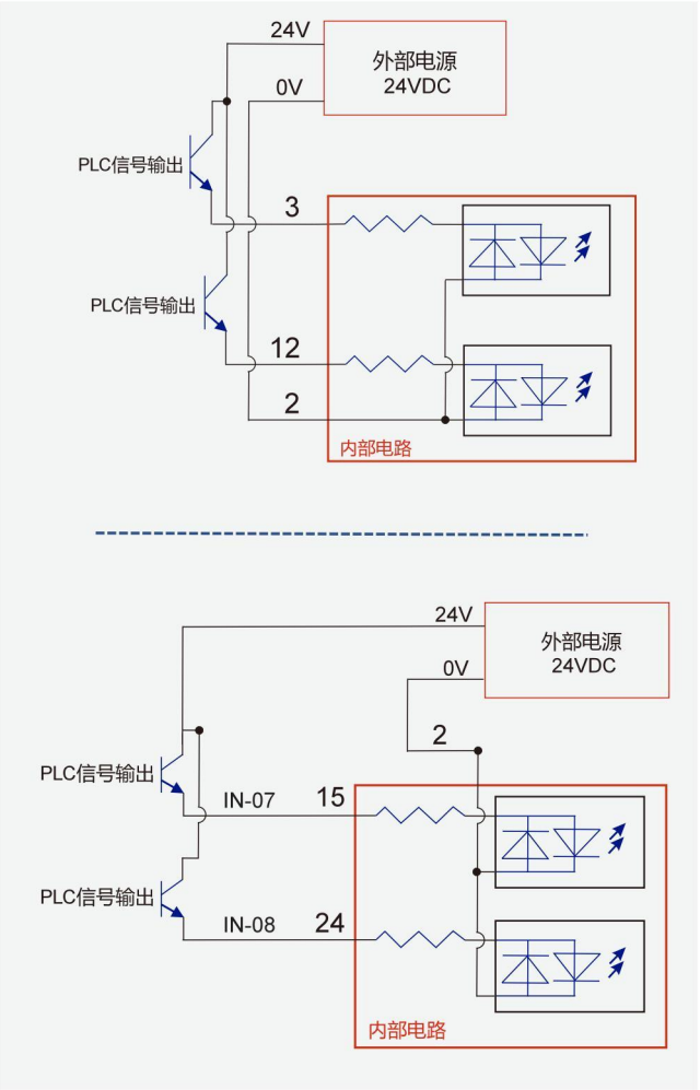
图 2-10：示教输入 IO 与 PLC 接线图
