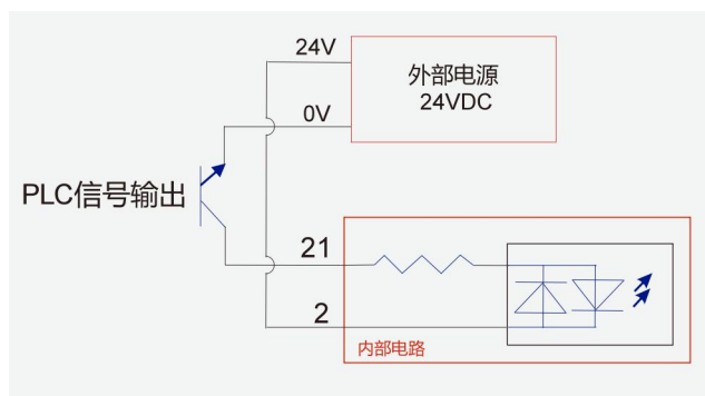
NPN（漏型）接法
