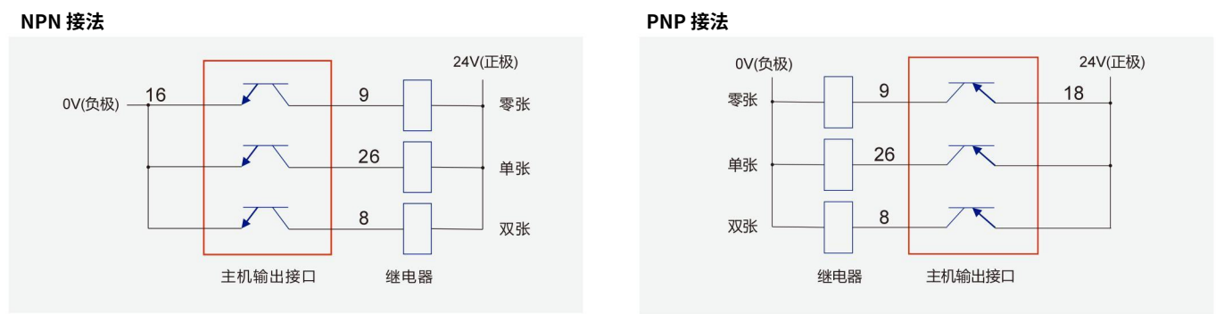
图 2-7：主机输出接口与继电器接线图
