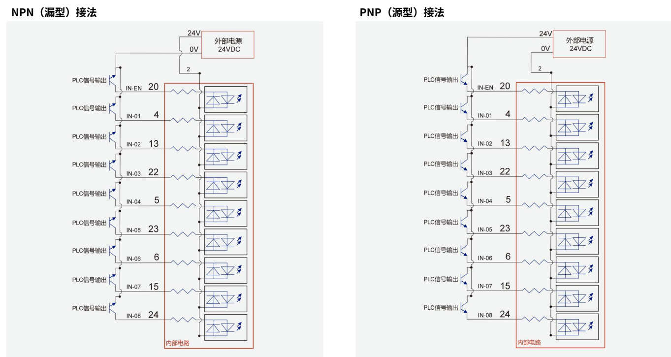
图 2-9：外部 IO 选择片料组别接口与 PLC 接线图
