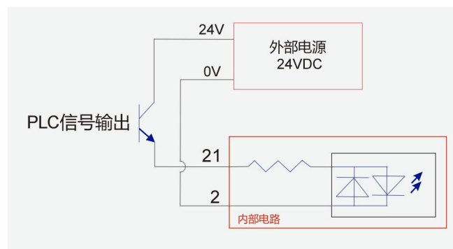
PNP（源型）接法
