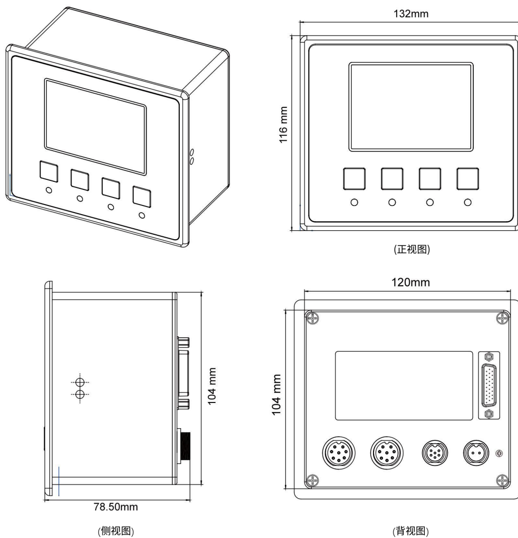
图 1-1: 主机尺寸图
